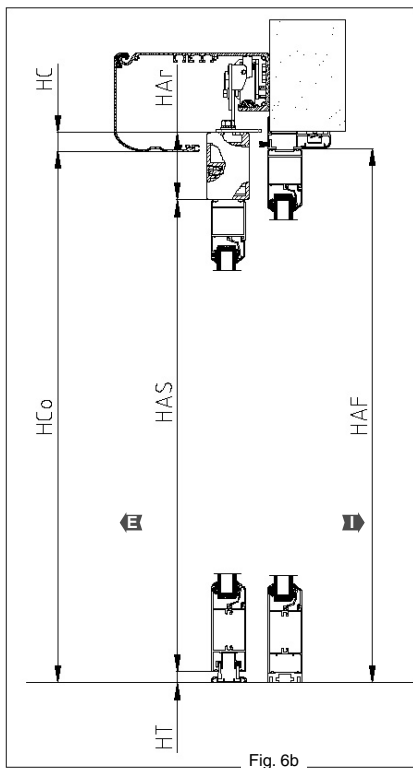
Serramenti SESAMO Magnum (Fig. 6b)
