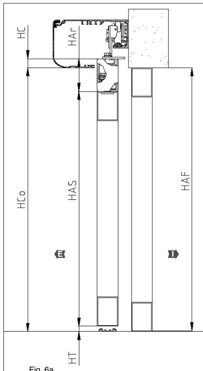
Serramenti Standard (Fig. 6a)
