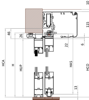
Section Magnum avec partie fixe
