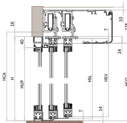
Section télescopique S30
