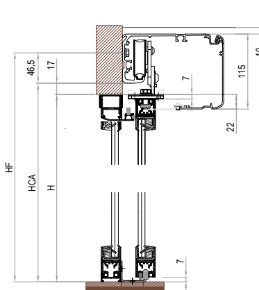
Section S30 avec partie fixe
