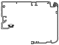
Profilé caisson légère
