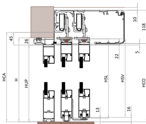
Section télescopique Magnum
