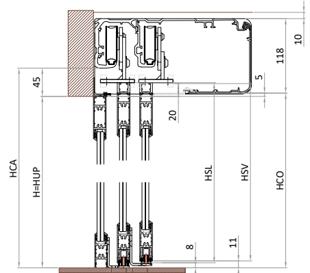
Section télescopique Twenty
