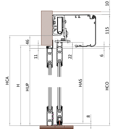
Section Twenty avec partie fixe
