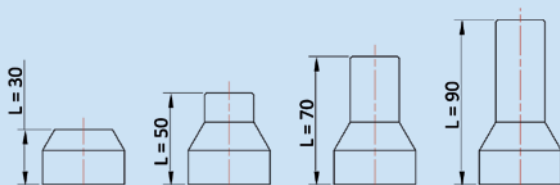
Rallonge bras en 4 mesures ART0332 / ART0333 / ART0334 / ART0335
