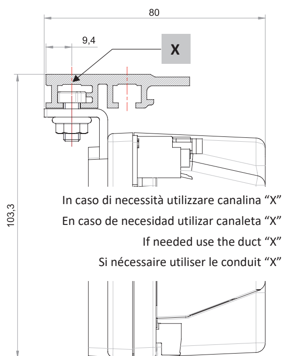
Sez. Modulo Centrale Elettronica / Secc. Modulo Centralita electronica Control Board Section / Section de la platine electronique
